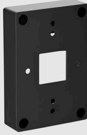
OMEGA HID SE İçin Sıva Üstü Reader Kasası 118 x 80 x 25 mm
