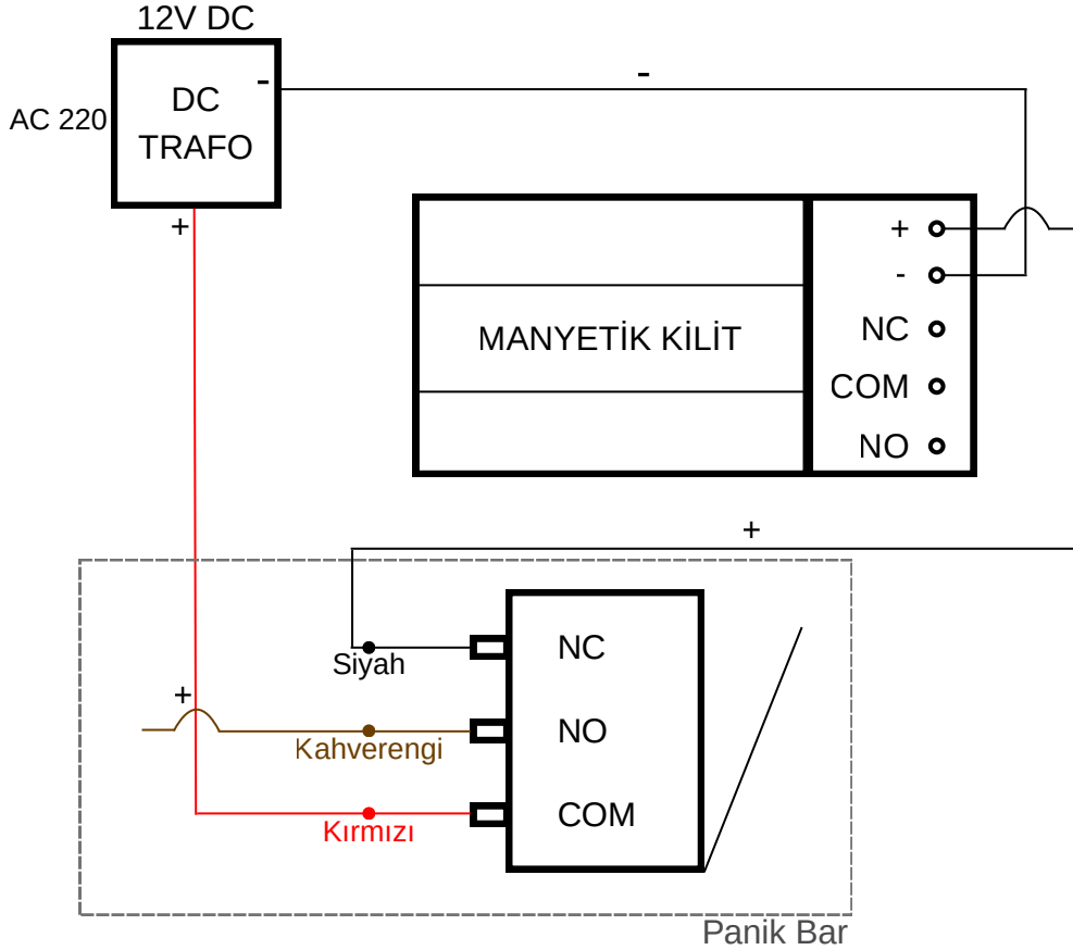
Manyetik Kilit - Panik Bar Bağlantı Şeması
