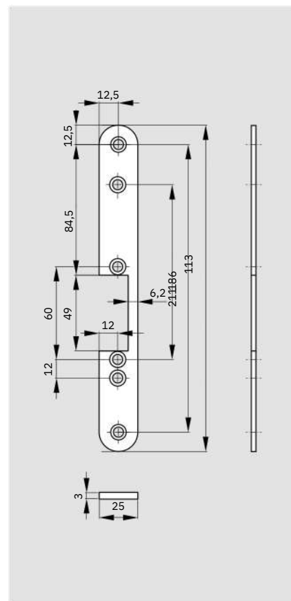
FKR 505/506 25-210
