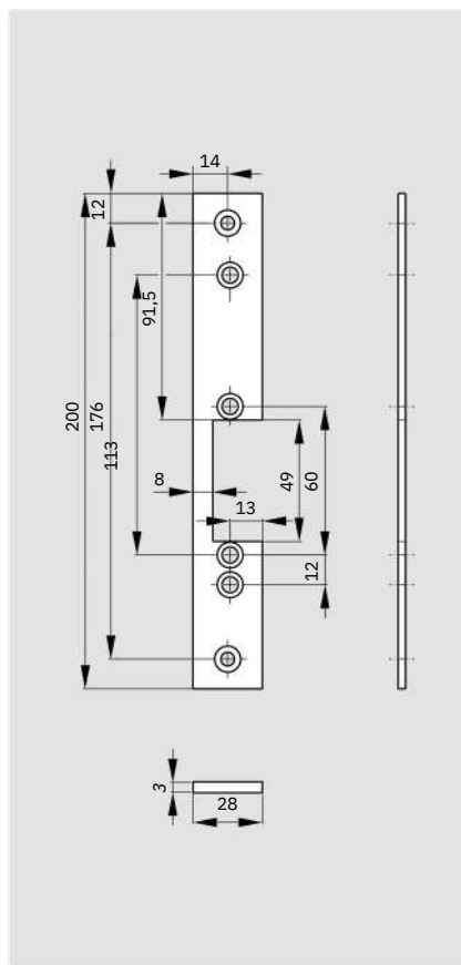
FKM 505/506 28-200
