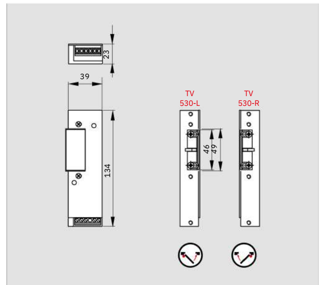
TV 530
