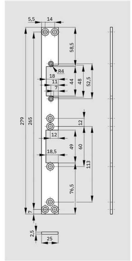
FKM 530 25-280
