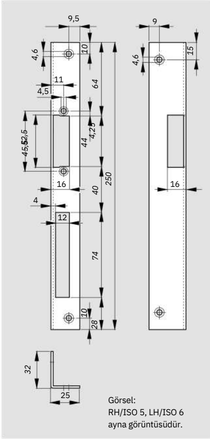
WR 25 / WL 25
