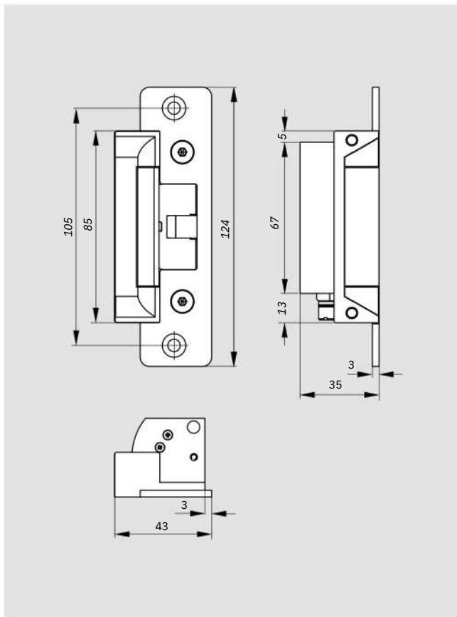
DES 300
