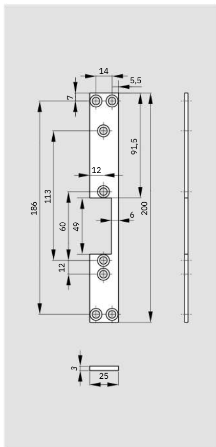
FKM 505/506 25-200
