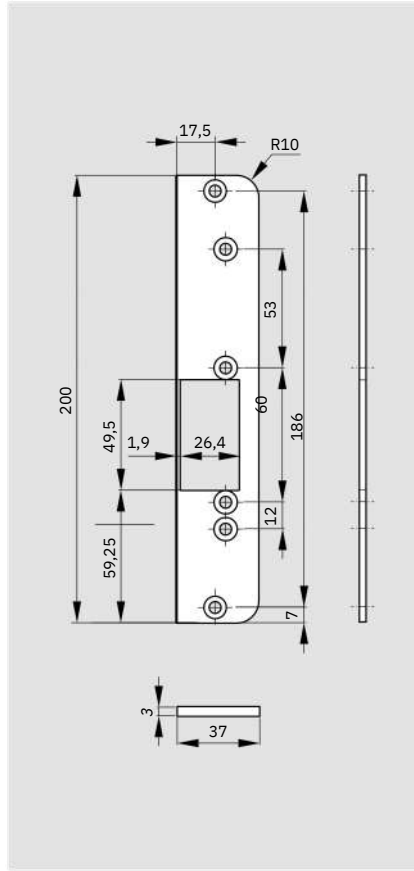
FK 507/508 37-200
