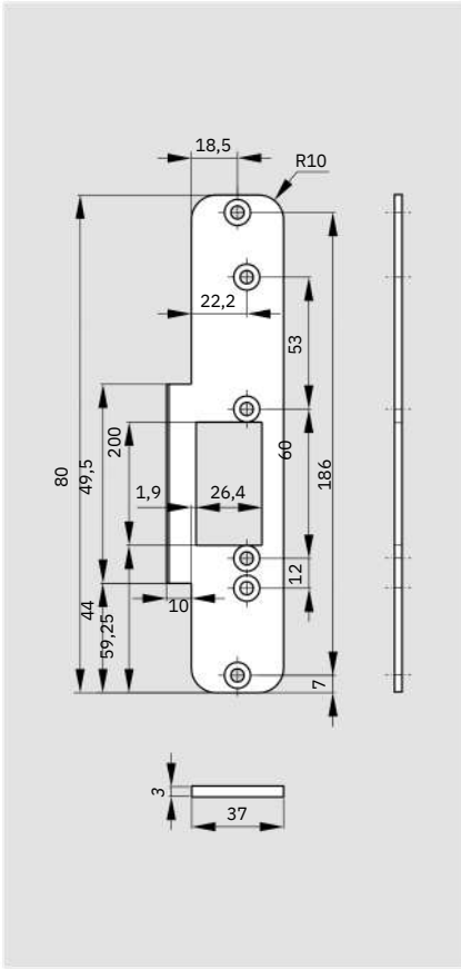
FKR 507/508 37-200
