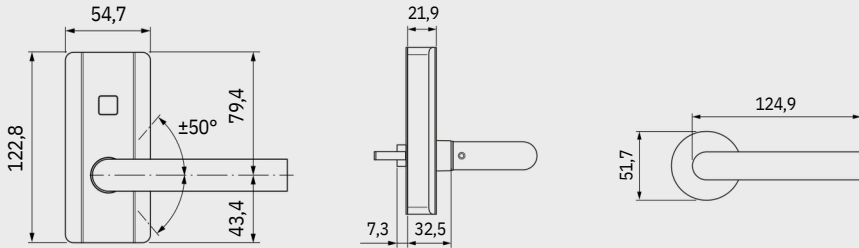
C-kollu kompakt, standart versiyon. Tip 2725
