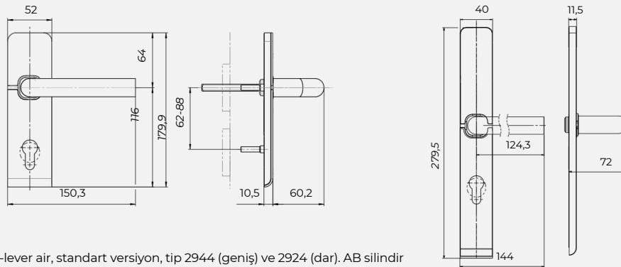
c-lever air, standart versiyon, tip 2944 (geniş) ve 2924 (dar). AB silindir profillerinin (kesikli çizgi) ve İsviçre yuvarlak profillerinin (kesikli çizgi) gösterimi.
