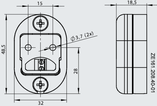
Dormakaba kayıt ünitesi 90 03'ün çizimi (Ölçüler mm cinsinden).
