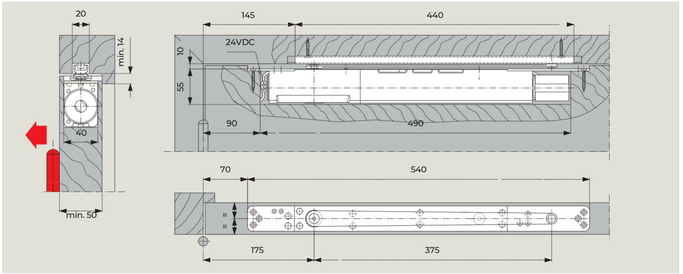
Ahşap bir kapıda G 96 N20 sürgülü kanala sahip ITS 96 İngiltere standardı mil FL kapı kapatıcısı. Örnek: Saat yönünün tersine kapanan (ISO 6) kapı; ayna görüntüsü saat yönünde kapanan (ISO5) kapılar için de geçerlidir.
