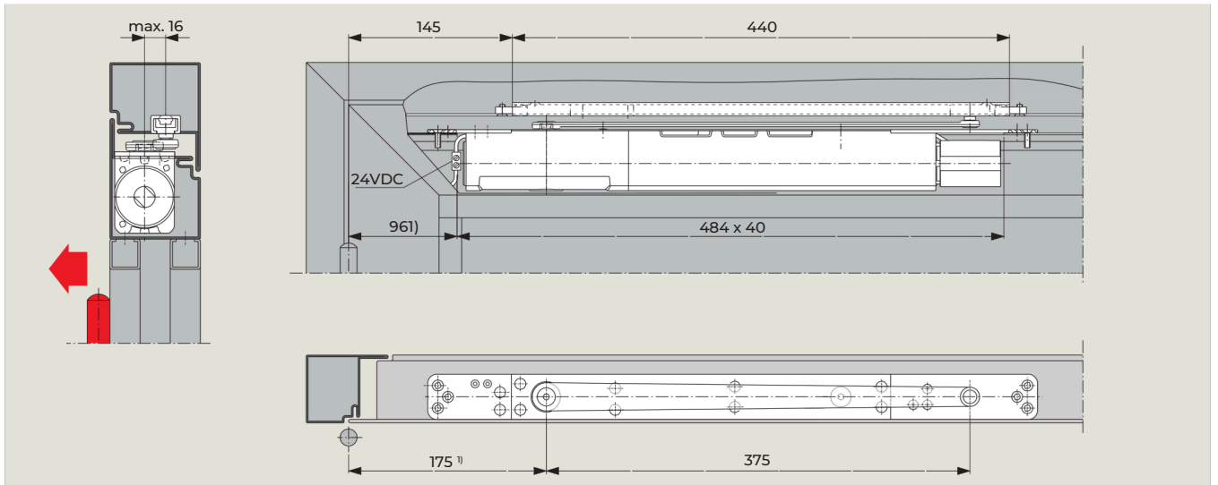
Alüminyum çerçeveli bir kapıda G 96 N20 sürgülü kanala sahip ITS 96 FL kapı kapatıcısı. Örnek: Saat yönünün tersine kapanan (ISO 6) kapı; Ayna görüntüsü saat yönünde kapanan (ISO 5) kapılar için geçerlidir.
