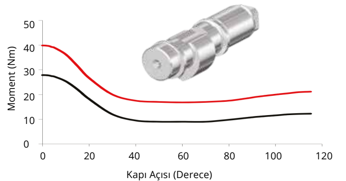
ITS 900 kam mekanizmalı kapı kapatıcısının (Boyut 4) moment profili
