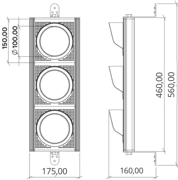
Ölçü Birimi: mm Şekil 4.6 – TRFL3 ölçüleri.
