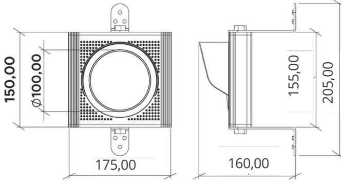
Ölçü Birimi: mm Şekil 4.4 – TRFL1 ölçüleri.
