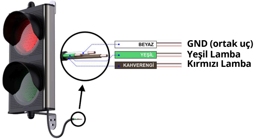
Şekil 3.2 – TRFL2 Bağlantı Şeması
