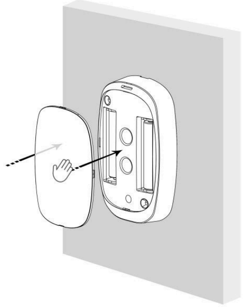
Ön plastik cam takılır
