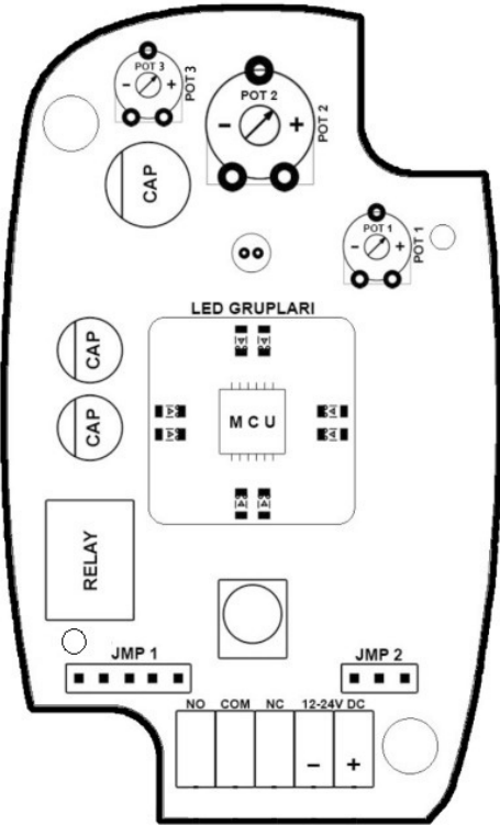
Şekil 1 – El Sensörü Kontrol Kartı
