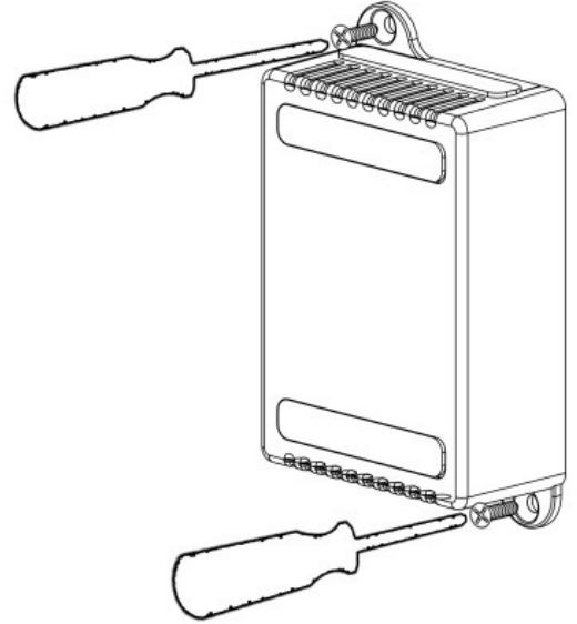
Şekil 7 - Duvara Montaj
