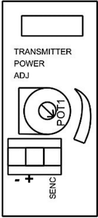
Şekil 1 - Verici Modül
