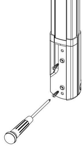
Şekil 5 - Vidaların Açılması
