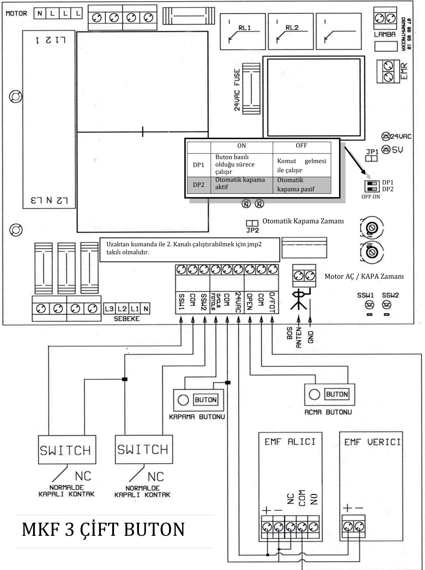
Şekil 1- MKF3 Çift Buton Bağlantı Şeması
