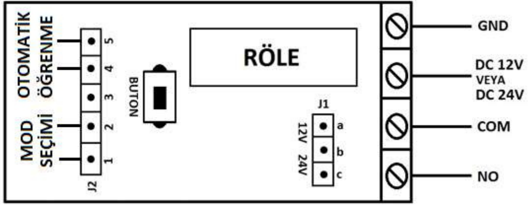
Şekil 6 - MKA Üstten Görünüş
