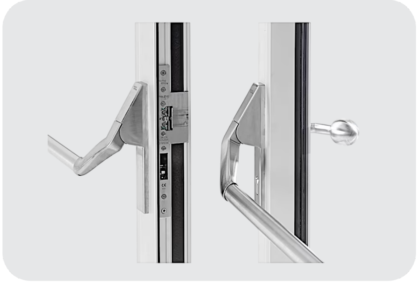
DORMAKABA PHA 2500 - Naturel Gömme Tip Panik Bar Sistemi
