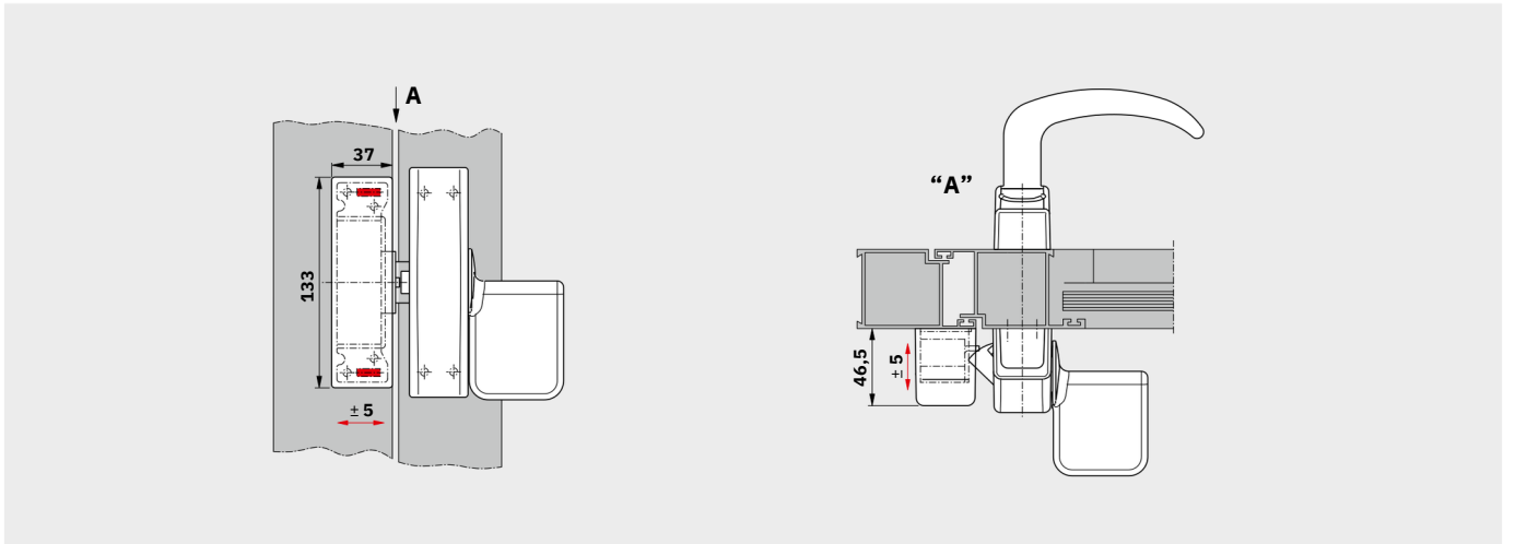
Alüminyum çerçeveli bir kapıda Exit Ped PHX 50 için uygulama örneği
