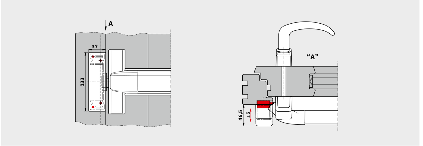
Ahşap bir kapıda PHX 50 ile PHB 3000 için uygulama örneği
