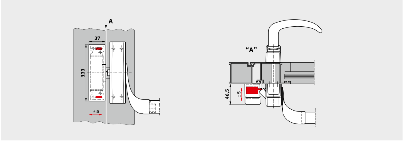
Alüminyum çerçeveli bir kapıda PHX 50 ile PHA 2000 için uygulama örneği
