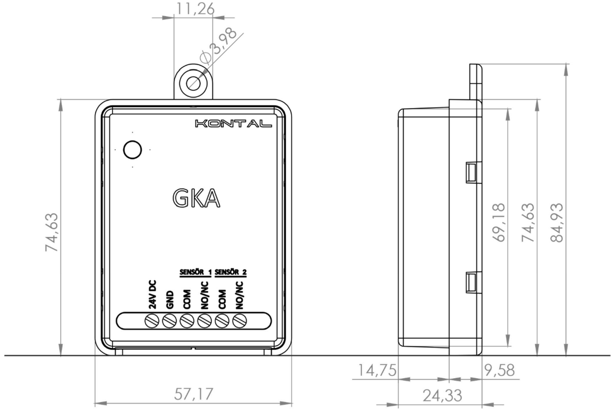
Şekil 16 - GKA Boyutlar
