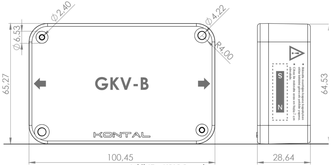
Şekil 17 - GKV-B Boyutlar
