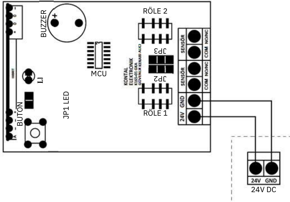
Şekil 12 - GKA Bağlantı Şeması
