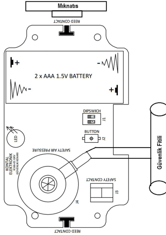
Şekil 11 – GKV-B Bağlantı Şeması
